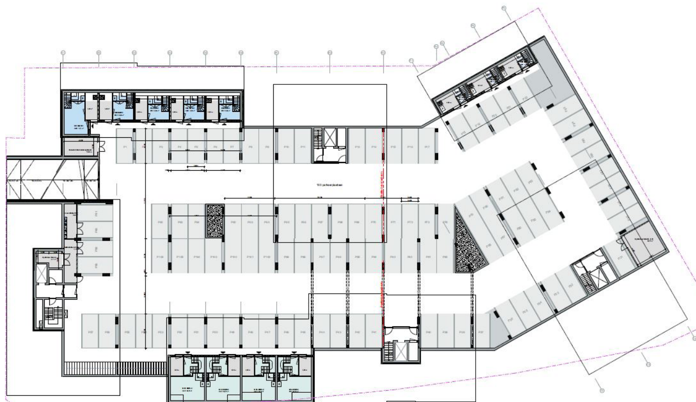
Afbeelding: Ontwerp parkeerkelder
