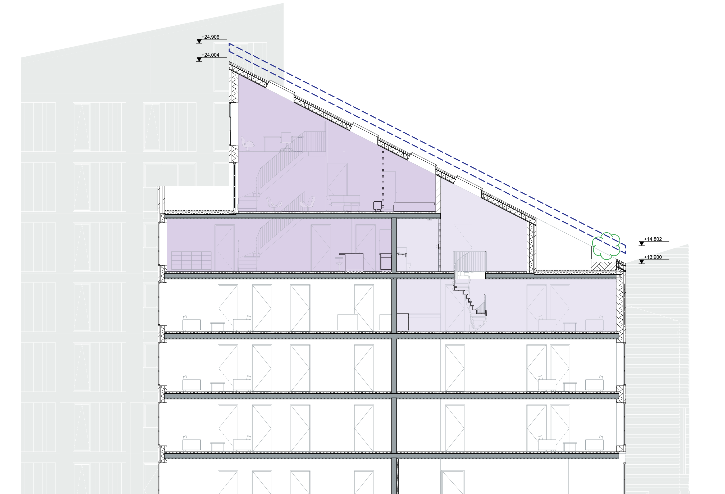
BLOK E | DOORSNEDE TOP VERDIEPINGEN | VOORSTEL
