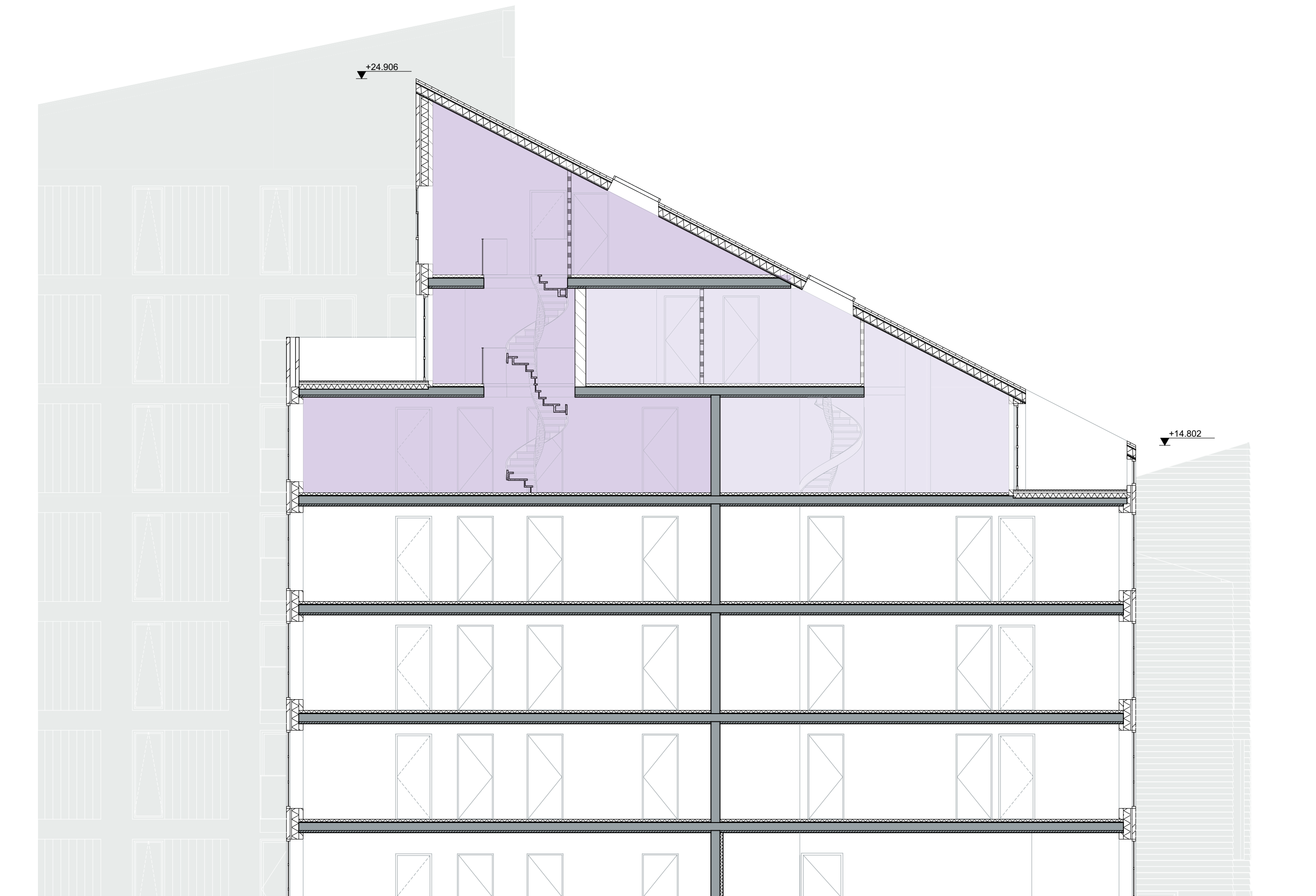
BLOK E | DOORSNEDE TOP VERDIEPINGEN | HUIDIGE SITUATIE
