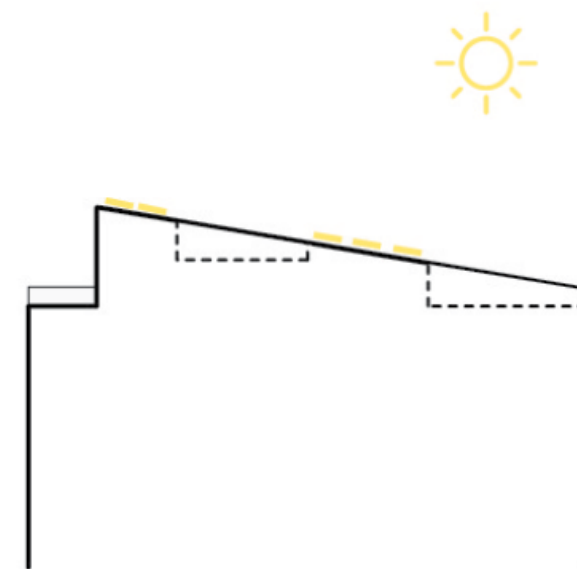
Afbeelding: Ligging tov waterkering
